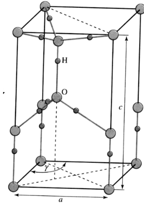
Maille élémentaire de la glace hexagonale (celle des glaçons, des flocons de neige...)
