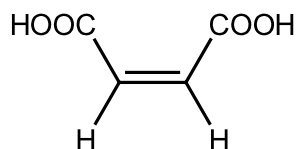
acide maléique
