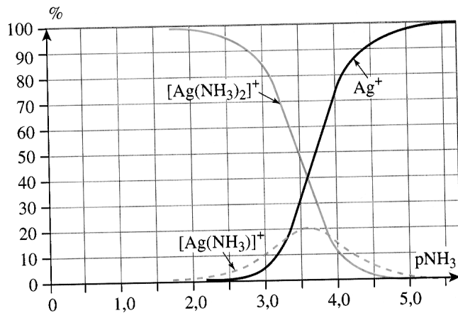
Diagrammes de distribution des complexes de l'ammoniac avec l'ion \text{Ag}^+ en fonction de \text{pNH}_3 = -\log [\text{NH}_3] . L'ion complexe [\text{Ag}(\text{NH}_3)]^+ n'est jamais l'espèce prédominante.
